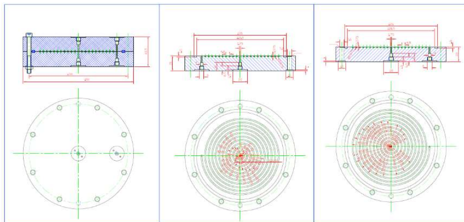
Ridicarea la scară a sistemului SLM de extracție și concentrare a pirazinelor
